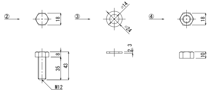
《 付属品 》
