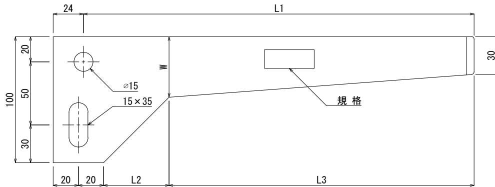
《 立面図 》
