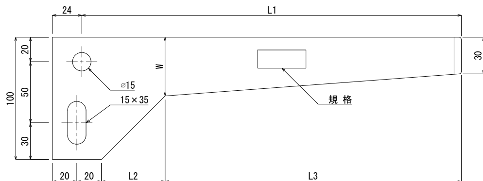
《 立面図 》
